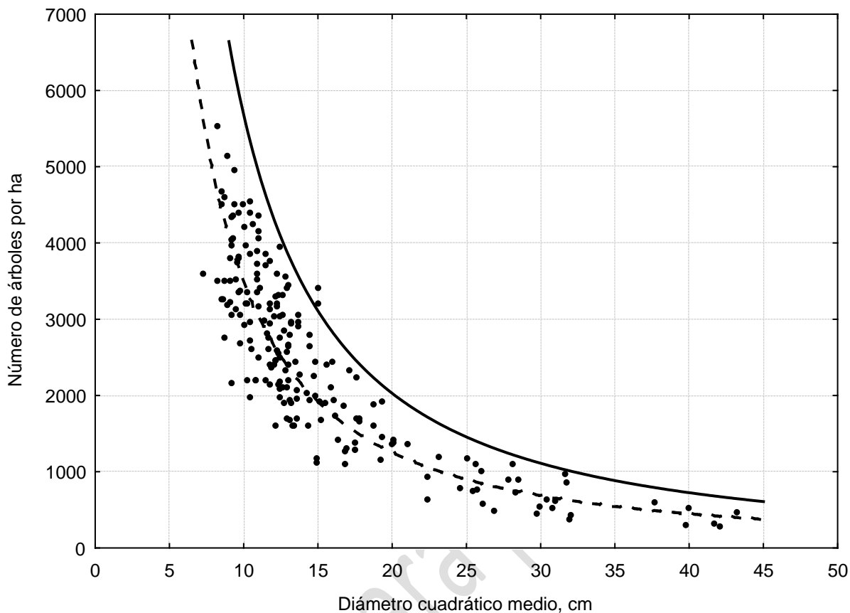
Figura 1. Ajuste del modelo de Reineke (1933) entre el número de árboles por hectárea y el diámetro cuadrático medio. Línea punteada: densidad promedio (ecuación [5]). Línea continua: densidad máxima (ecuación [6]).
