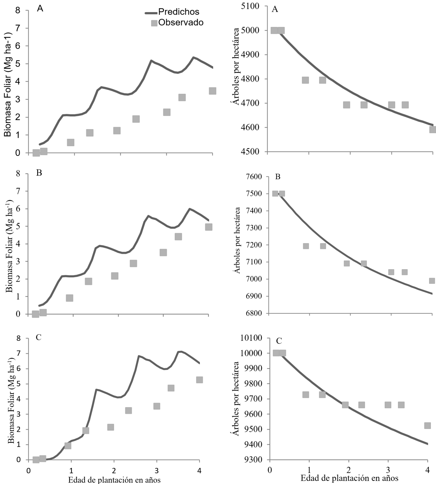
Figura 3. Resultados de la modelación en 3PG de la biomasa total de follaje (Mg ha -1 ) y Mortalidad (árb ha -1 ) para las densidades de 5000 (A), 7500 (B) y 10000 (C) árb ha -1 .
